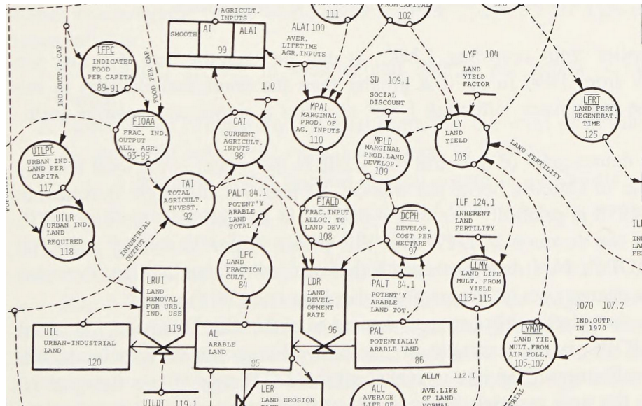
Figure 2: Extrait du diagramme d'influence mutuelle des variables pour le secteur de l'agriculture, tiré de la documentation technique [20]
