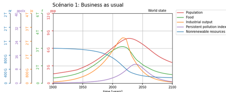
Figure 16: Usage de pydynamo pour le modèle World3
